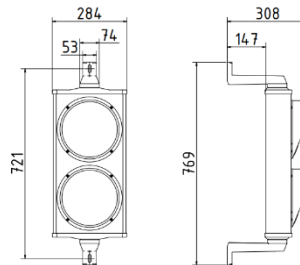
Helios 200 zweifach Ampel
