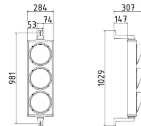
Helios 200 dreifach Ampel
