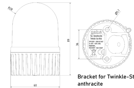
Twinkle-Star Mini 24V AC/DC Ref.: 905.MBSL.10 230V AC Ref.: 905.MBSL.20
