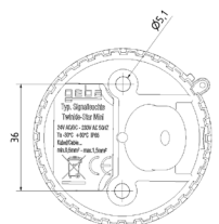
Bracket for Twinkle-Star Mini anthracite Ref.: 905.BWM1.00
