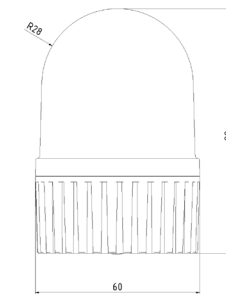
Twinkle-Star Mini 24V AC/DC Ref.: 905.MBSL.10 230V AC Ref.: 905.MBSL.20
