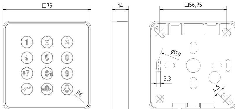
Cody Touch-Silber-Schwarz LED-Blau Art.: 507.BT21.03
